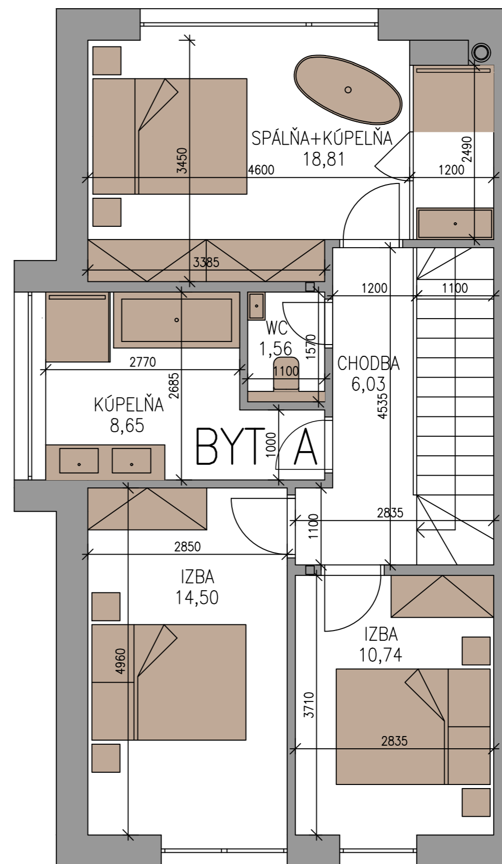
PÔDORYS 2.NP
